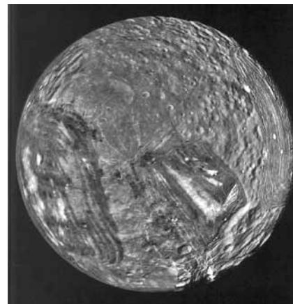
Uranusmånen Miranda viser både skrapemerker og andre anomalier etter ublide sammentreff med andre himmellegemer etter planetkatastrofen
