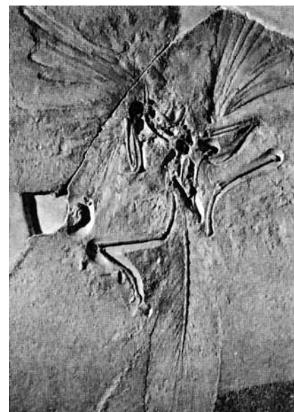
Berømt fossil av «urfuglen» Archaeopteryx
