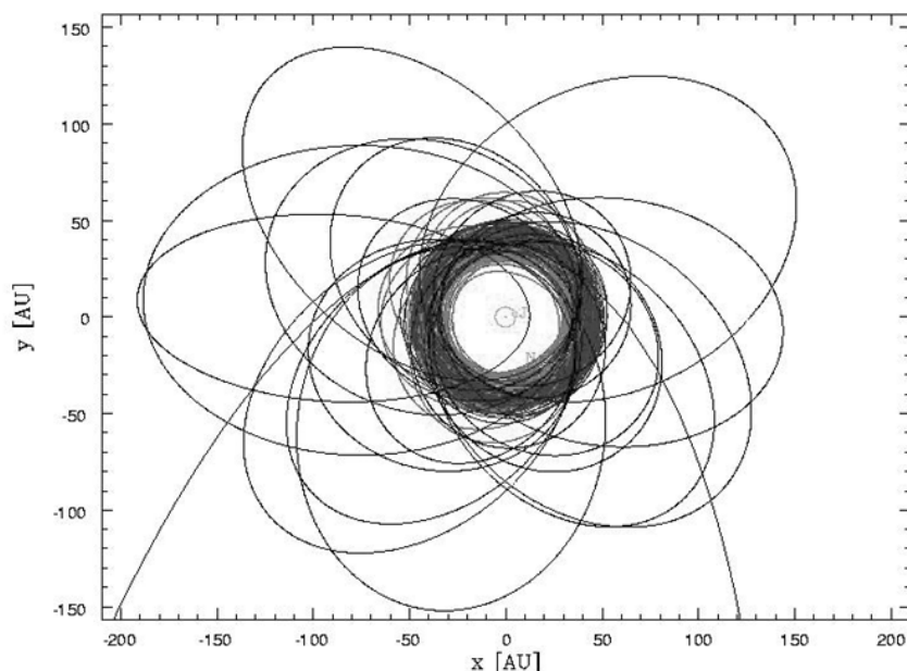
Kuiperbeltet utenfor Neptun kan inneholde så mye som 70 000 fragmenter etter en planetkatastrofe
