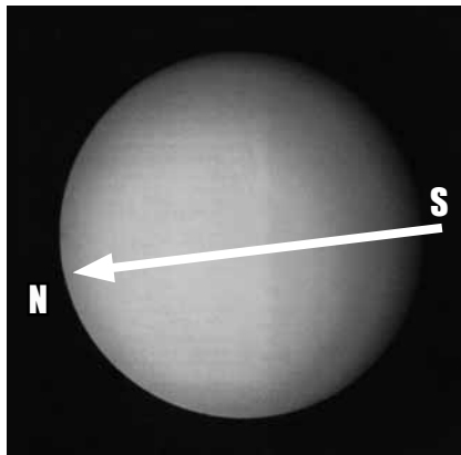
Rotasjonsaksen til Uranus er bikket kraftig over, og legger nesten vannrett i forhold til baneplanet
