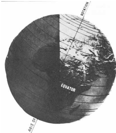
Jordas rotasjonsakse danner i dag en vinkel på 23^{\circ}26' i forhold til normalen
