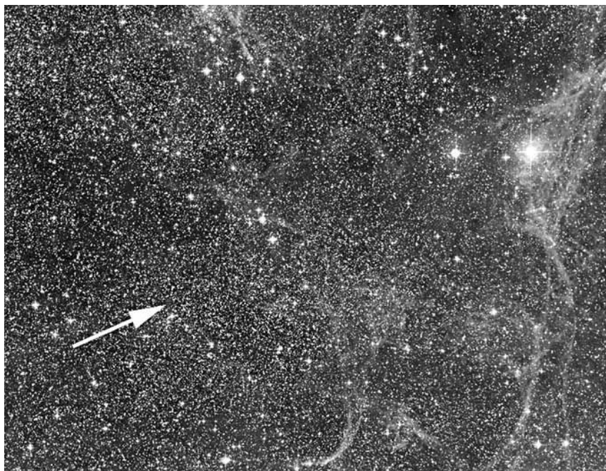
Restene etter supernovaen i stjernebildet Vela Pilen viser hvor pulsaren etter den eksploderte stjernen befinner seg
