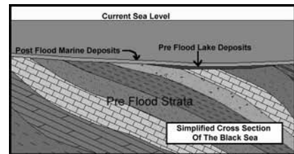
Strata under bunnen av Svartehavet
