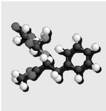
Modell av Aspartam-molekyl ( C_{14}H_{18}O_5N_2 ) L-asparti-L-fenylalanin metylester
