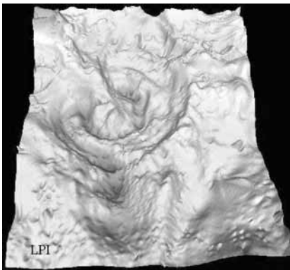
Chixculub-krateret på Yucatanhalvøya ved Mexicogulfen har en diameter på rundt 200 km og ble skapt av en asteroid med diameter på ca. 10–15 km
