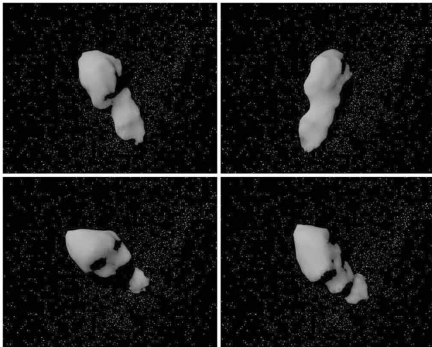
Asteroiden Toutatis sett fra flere vinklinger
