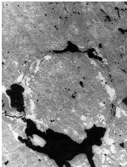
Siljan-krateret i Sverige har en diameter på 52 km
