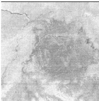
Popigai-krateret i Russland har en diameter på 100 km
