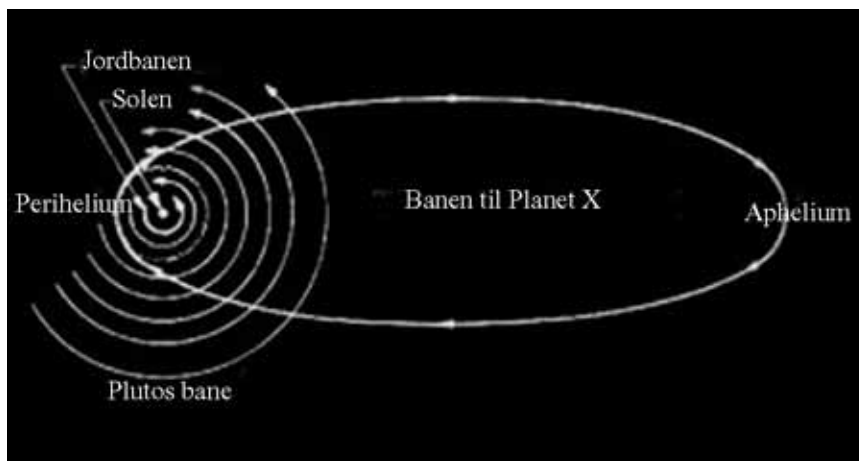
Skisse av banen til Planet X, slik astronomene tenker seg den. Det usikkerhet om banens aphelium (fjerneste punkt fra sola). Tallene varierer fra 50 til 25 000 Astronomiske enheter fra sola. Sikkert er det i hvert fall at banen strekker seg langt
